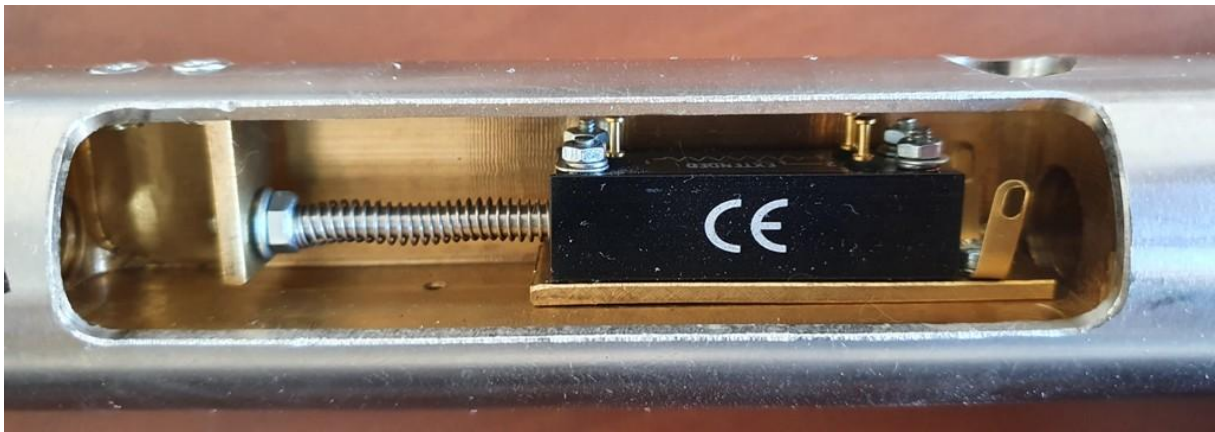
KGCT-3-80-43D lineáris potenciométer
